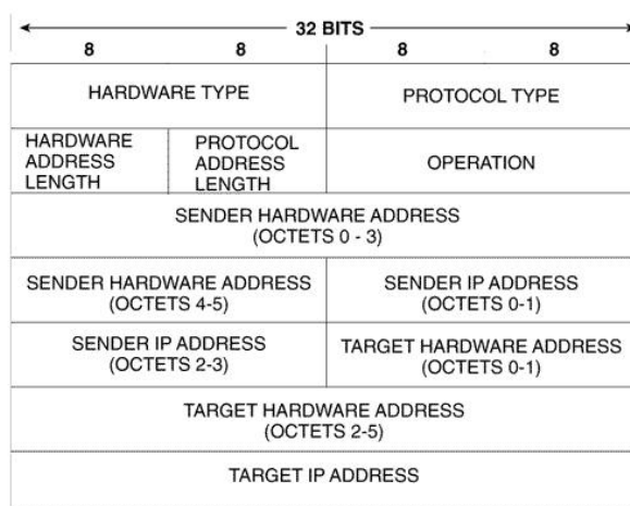
фигура 16. Заглавна част на ARP
