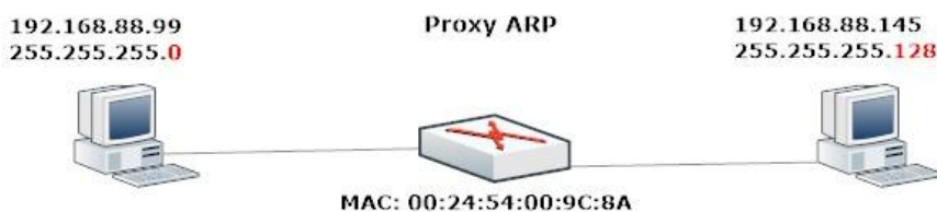
фигура 23. Proxy ARP
