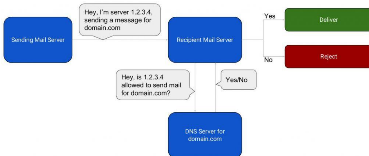
фигура 49 Схема на процес по SPF валидация
