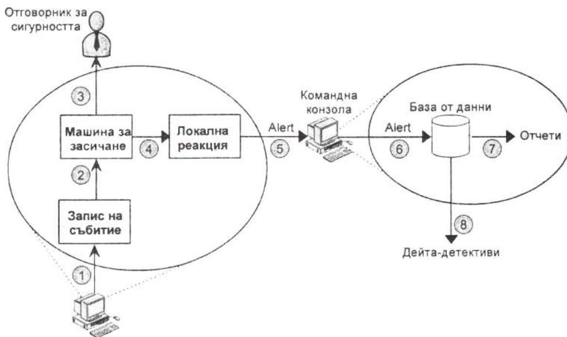
фигура 41. Разпределената архитектура в реално време
