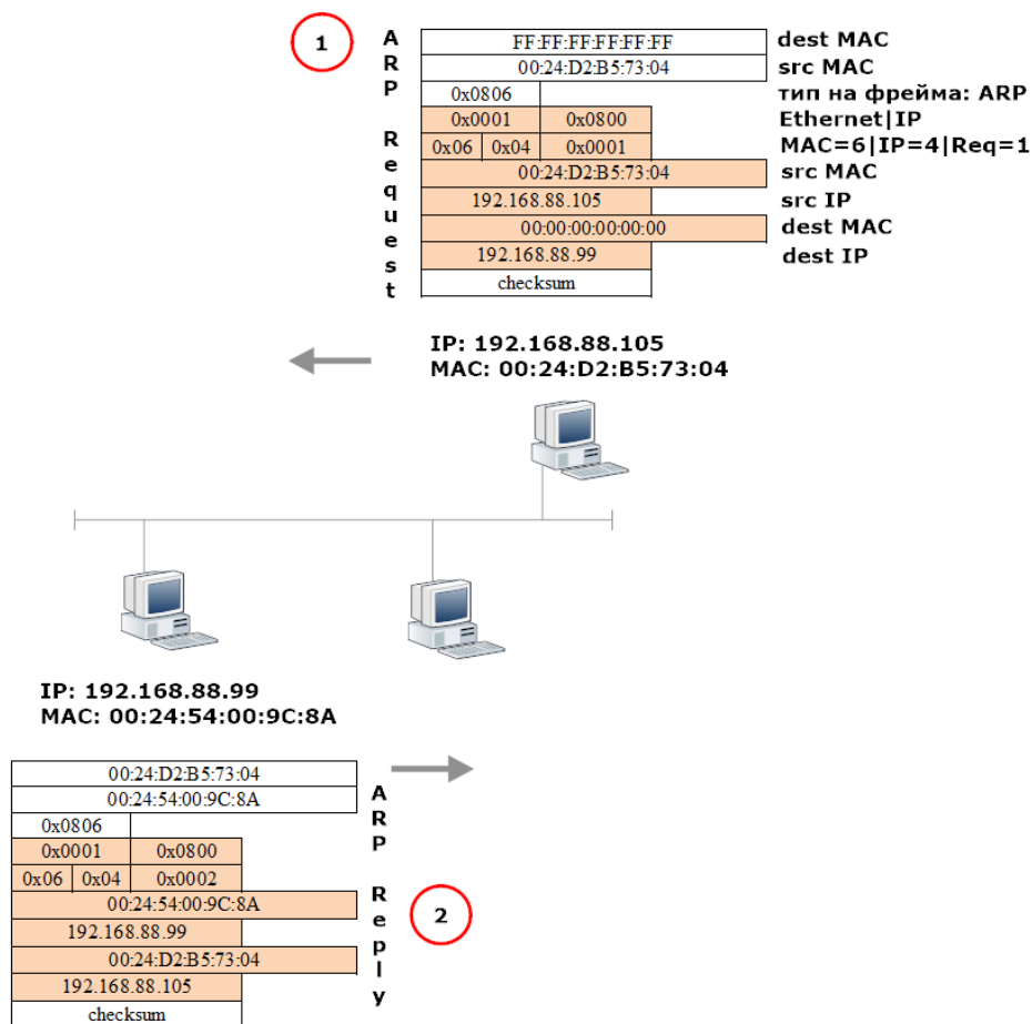
фигура 18. ARP заявка и отговор
