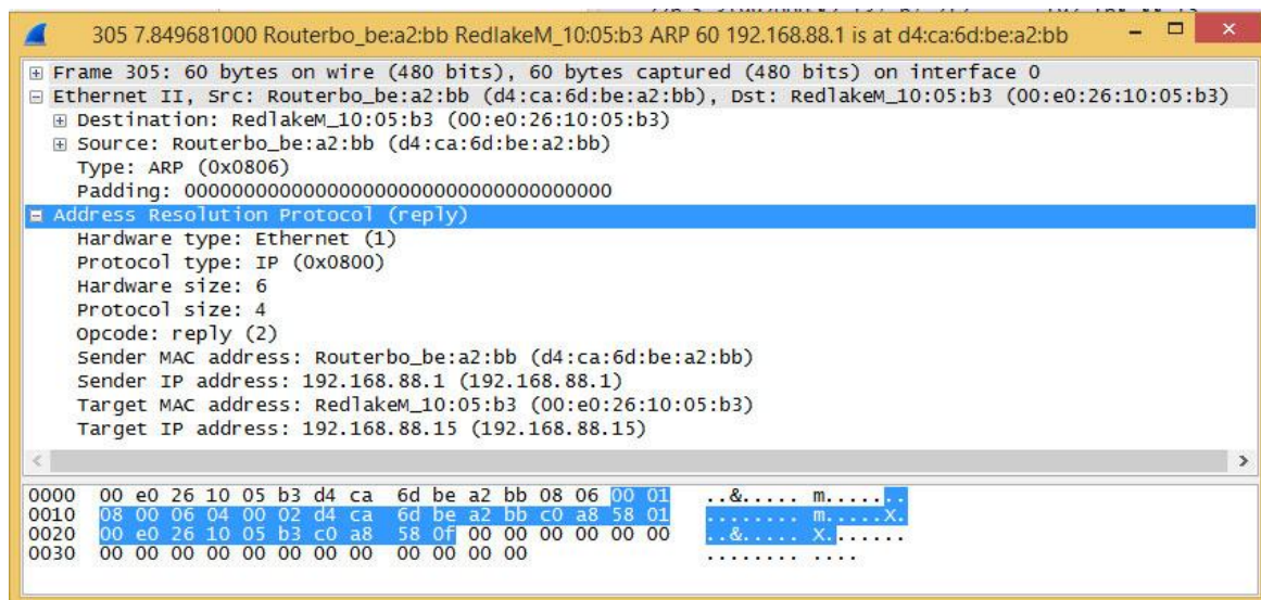
фигура 20. ARP отговор
