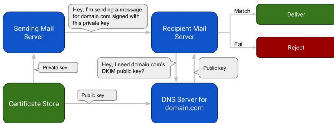
фигура 50 Схемa на процес по DKIM валидация
