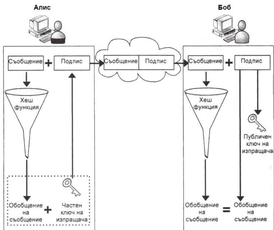
фигура 48 Процеса на създаване на RSA цифровия подпис
