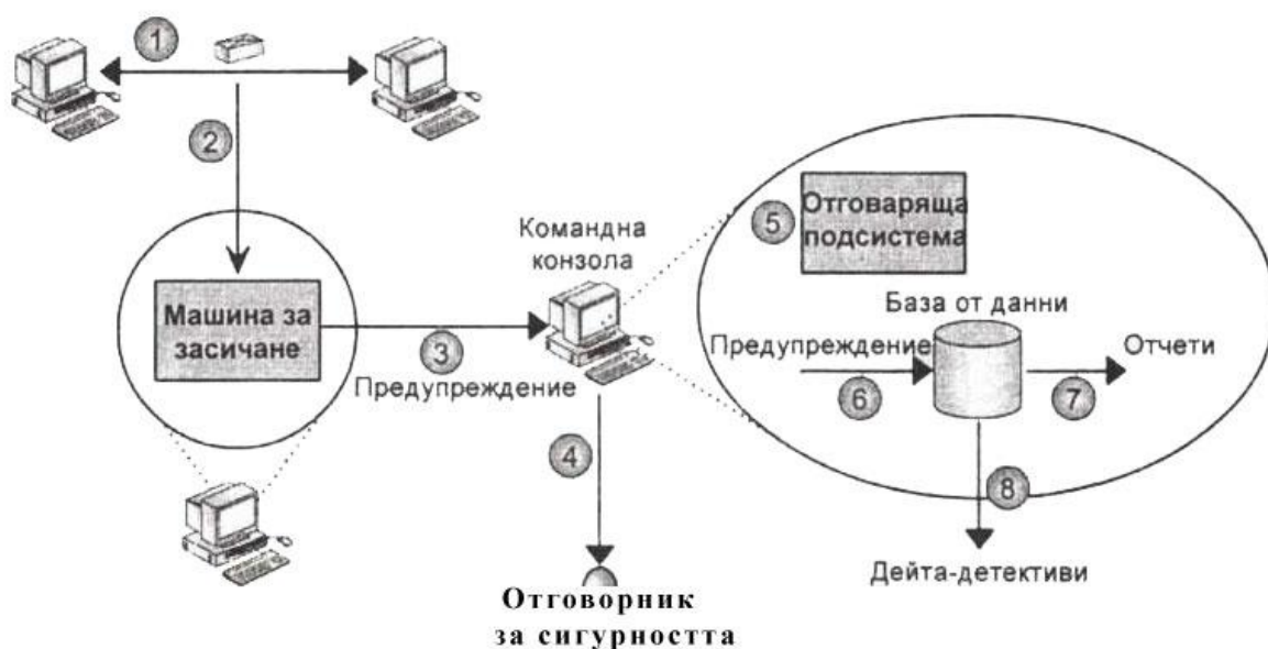
фигура 38. Традиционна мрежова архитектура
