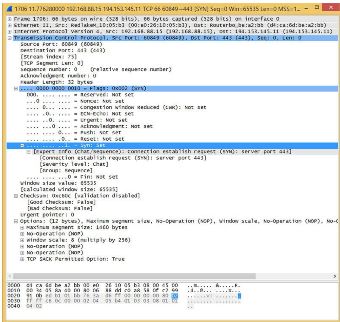
фигура 6. SYN сегмент
